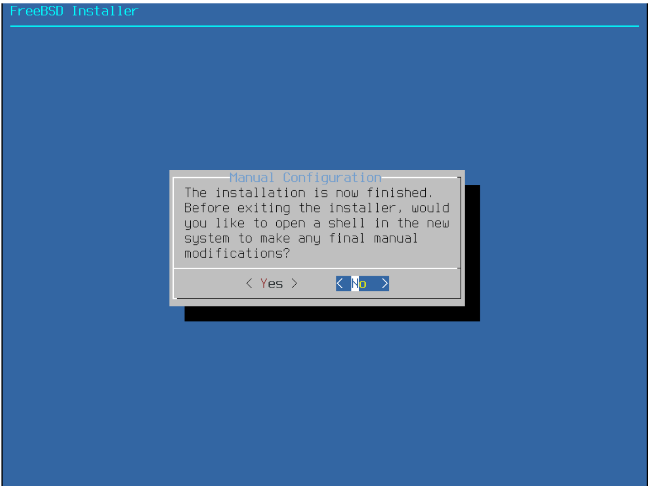
图 101. 手动配置
